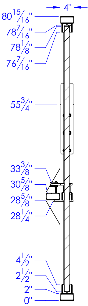
SECTION B-B SCALE 1 : 16
